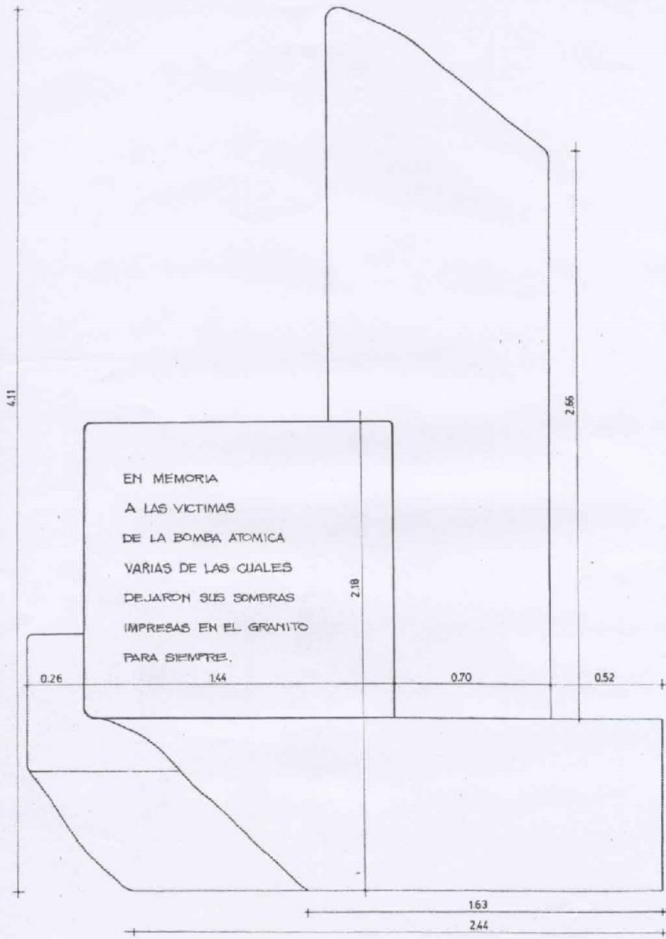
VISTA POSTERIOR.
