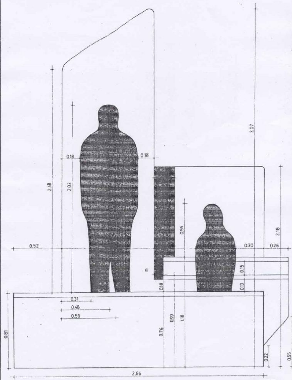
VISTA FRENTE
