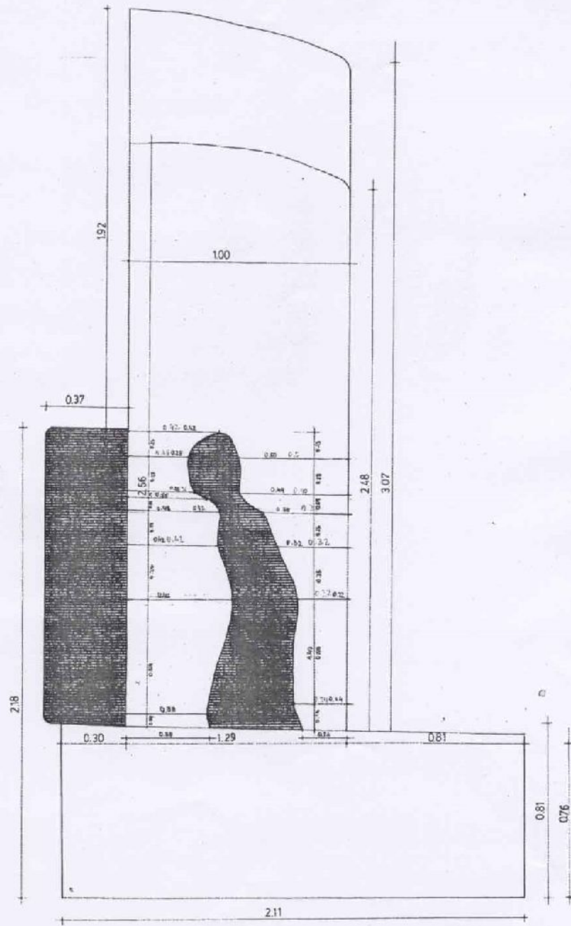
VISTA LATERAL IZQUIERDA
